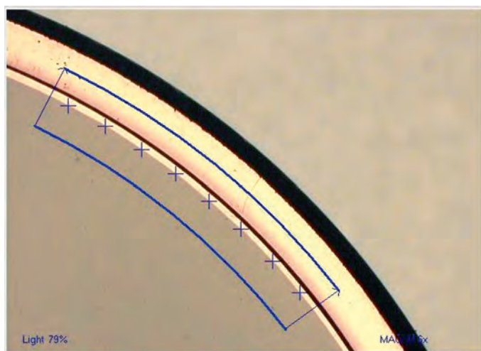
Mesure de couche de métallisation
