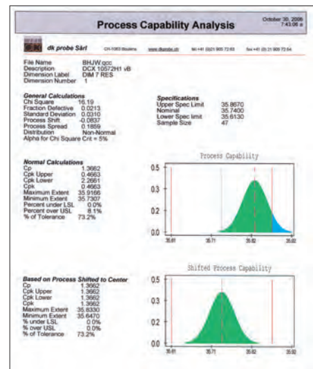
Analyse de capacité
