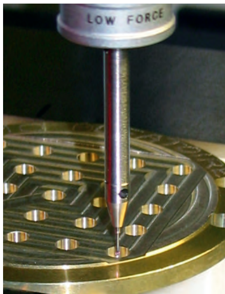
Mesure de pièces test processus de fabrication
