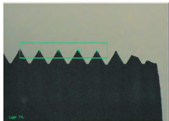
Mesure de filetage
