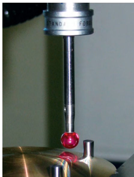
Mesure de gabarit
